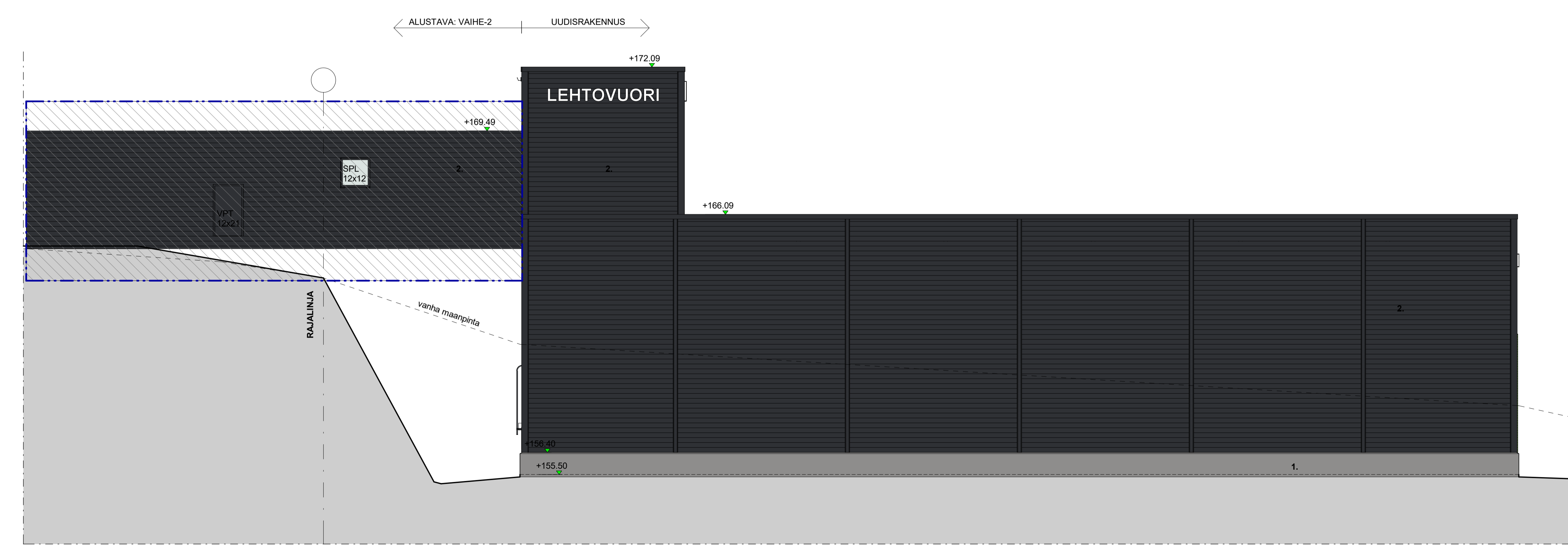
JULKISIVU KAAKKOON / HOPEATIELLE 1:100
