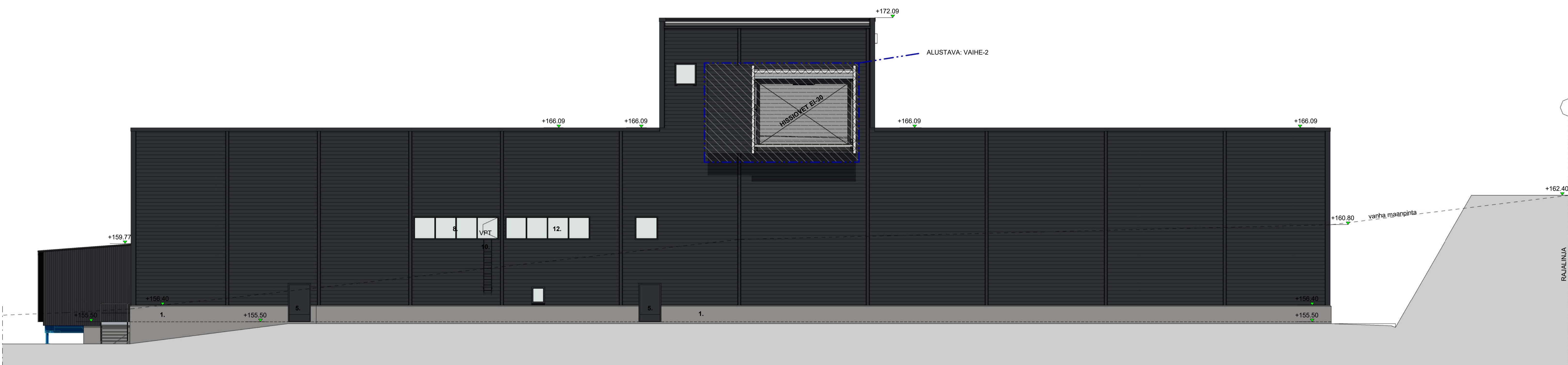
JULKISIVU LOUNAASEEN 1:100
